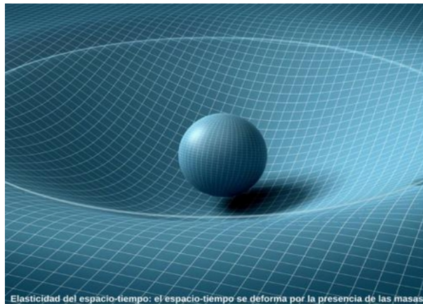
17. Elasticidad del espacio-tiempo por la presencia de las masas.
