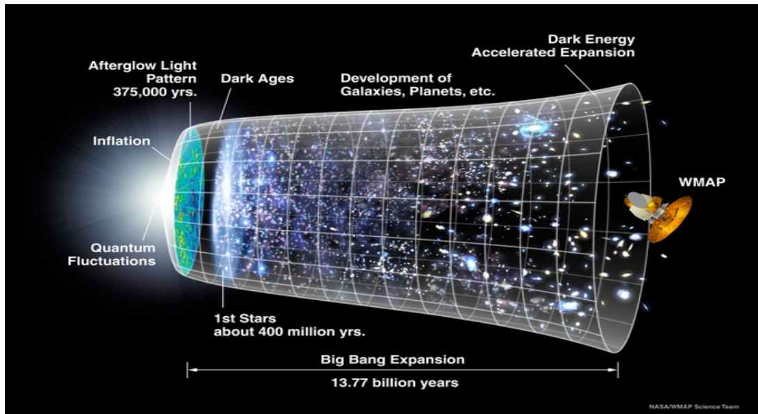
11. Representación actual de la evolución universal - NASA/WMAP Science Team. 17
