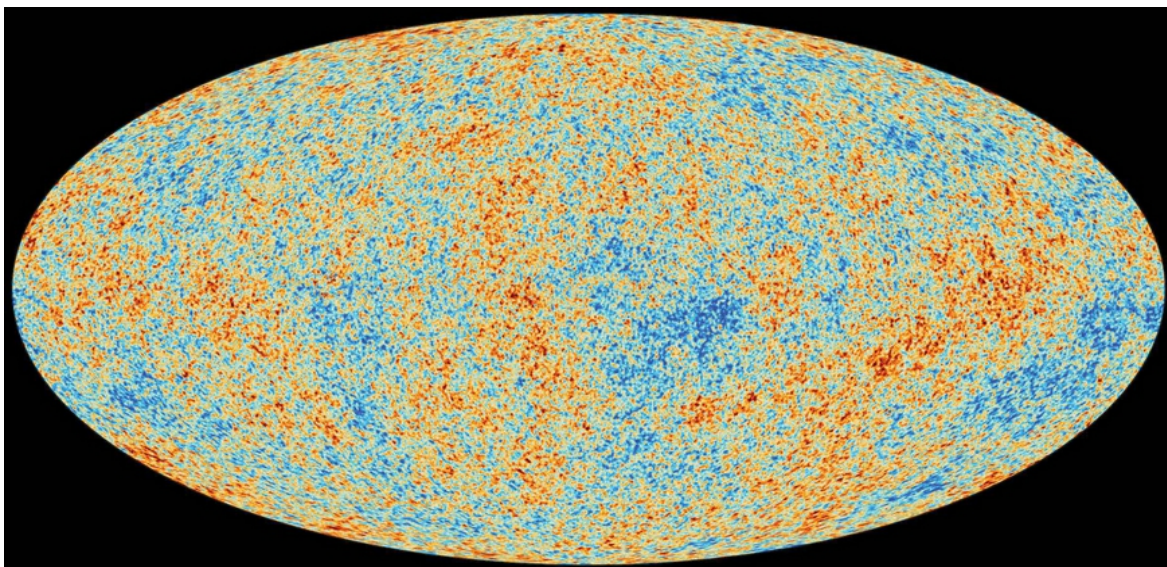
13. Radiación de fondo de microondas – Planck, ESA, 2013. 20
