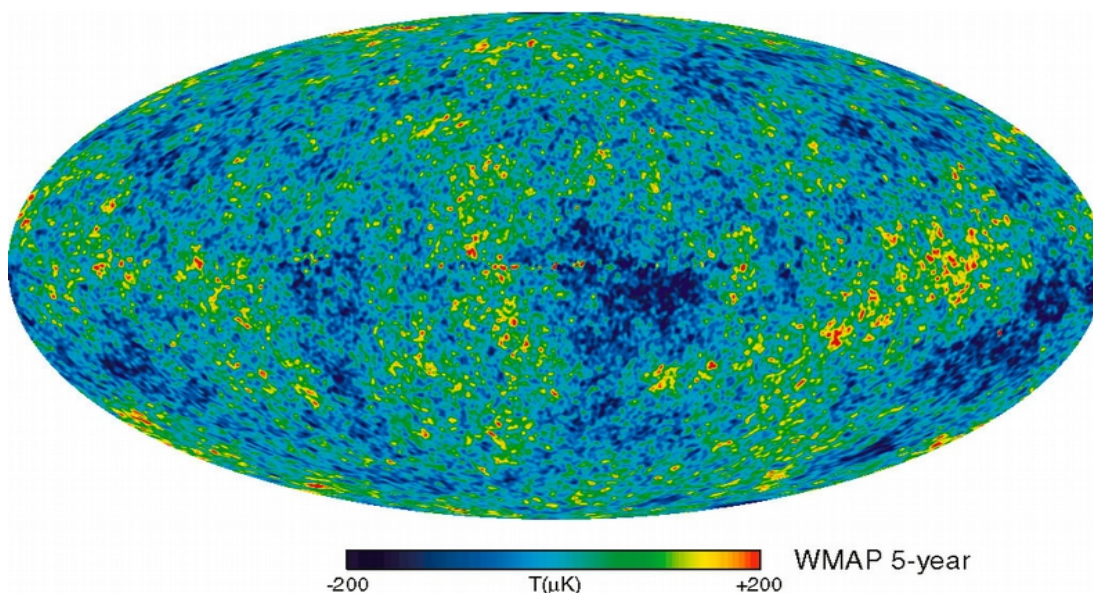
12. Radiación de fondo de microondas - NASA/WMAP Science Team, 2001. 19
