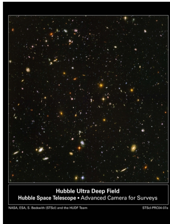
7. Campo Ultraprofundo de Hubble 12
